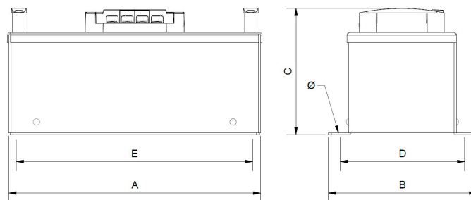
Dimensiones (AxBxCxDxE): 350x200x170x170x325 mm 6 
