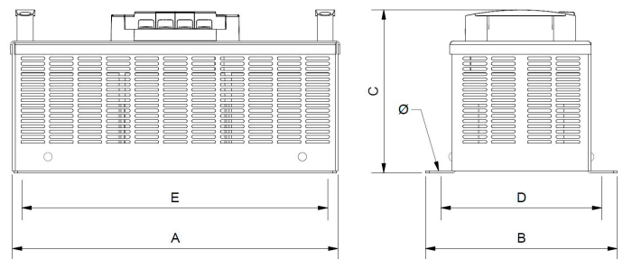
Dimensiones (AxBxCxDxE): 350x200x170x170x325 mm 6φ
