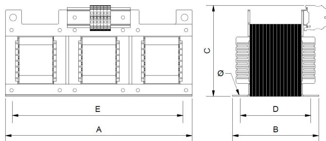
Dimensiones (Ax BxCxDxE): 325x160x170x130x295 mm 6Ø
