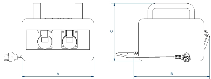
Dimensiones (AxBxCxDxE): 210x200x160 mm
