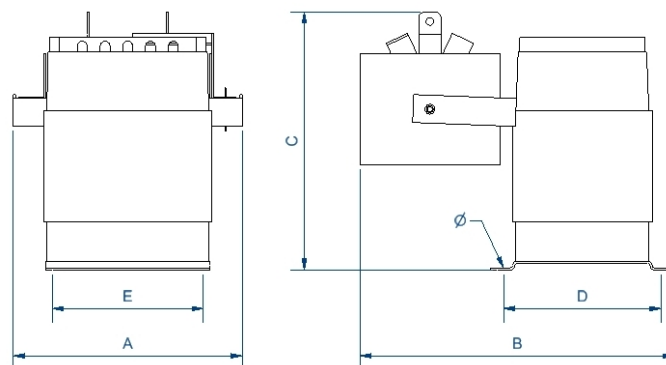
Dimensions (AxBxCxDxE): 240x290x200 mm 7Ø
