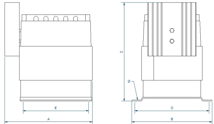
Dimensions (AxBxCxDxE): 167x145x191 mm 7Ø
