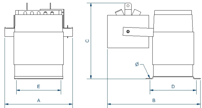
Dimensions (AxBxCxDxE): 240x290x200 mm 7Ø
