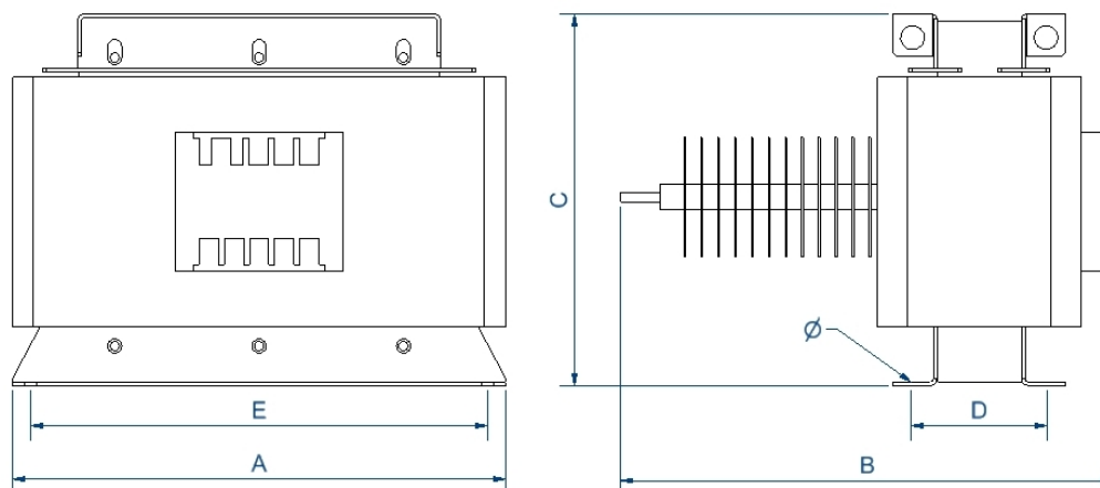
Dimensions (AxBxCxDxE): 238x195x205x177x150 mm 90°
