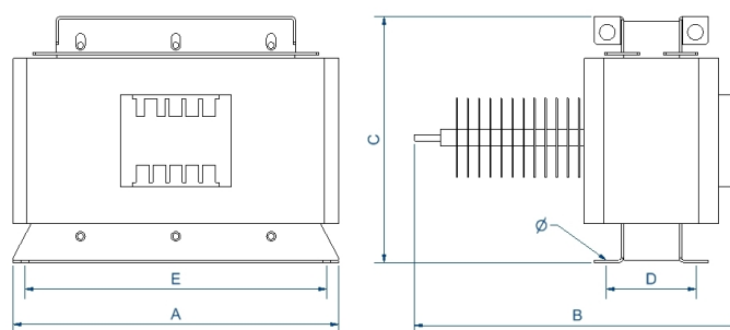
Dimensiones (AxBxCxDxE): 490x780x355x142x460 mm 11 
