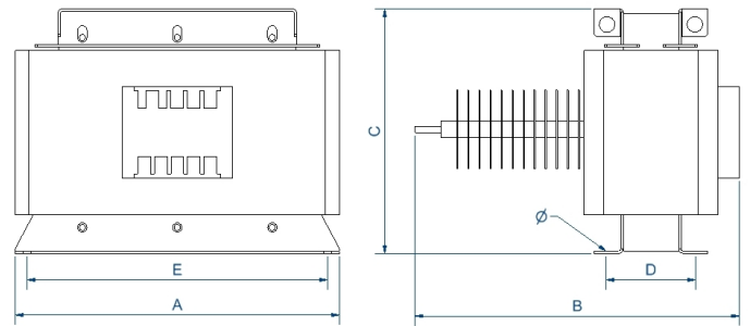
Dimensiones (AxBxCxDxE): 540x1090x405x164x510 mm 11 
