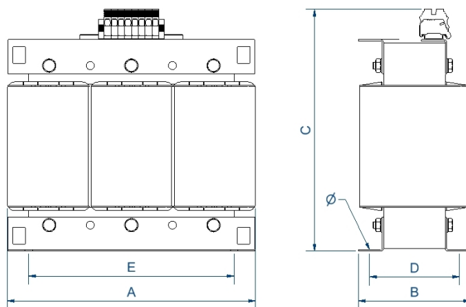
Dimensiones (AxBxCxDxE): 420x170x419x136x350 mm 11Ø
