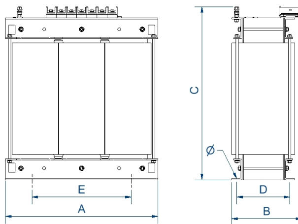
Dimensiones (AxBxCxDxE): 785x550x880x460x472 mm 17Ø
