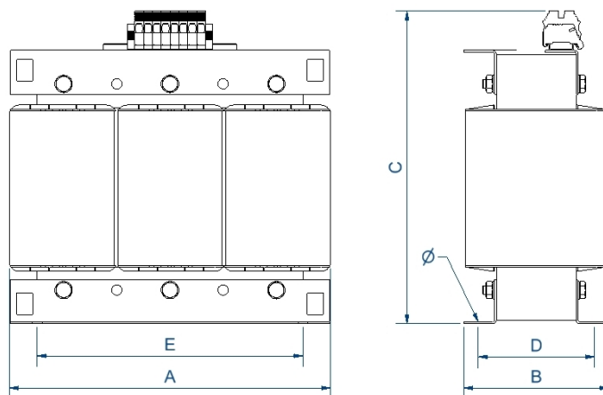
Dimensiones (AxBxCxDxE): 240x145x253x125x200 mm 9Ø
