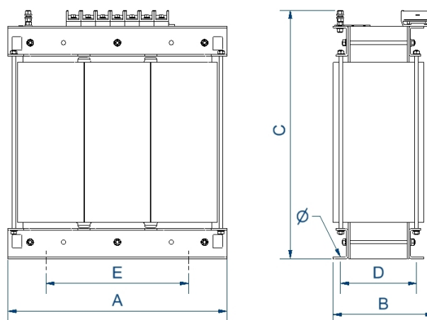
Dimensiones (AxBxCxDxE): 352x260x460x230x200 mm 11
