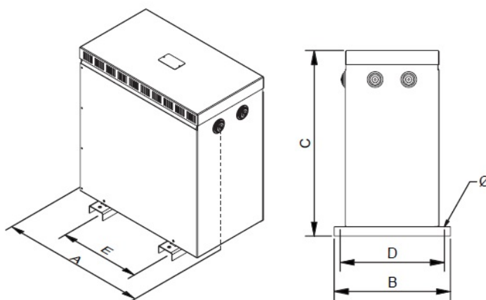
Dimensiones (AxBxCxDxE): 595x415x708x375x350 mm 12Ø
