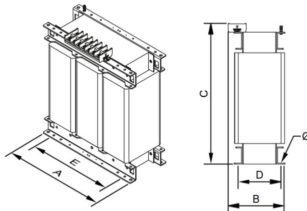
Dimensiones (AxBxCxDxE): 670x310x580x170x426 mm 13Ø
