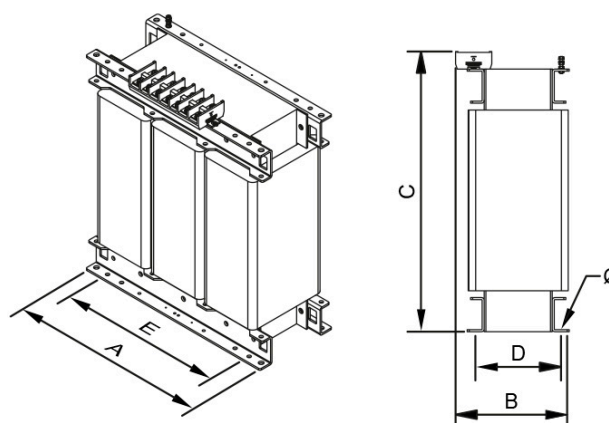
Dimensiones (AxBxCxDxE): 670x330x580x190x426 mm 13
