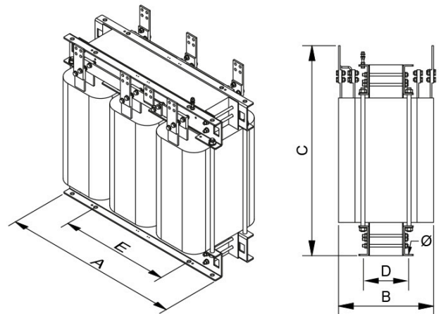
Dimensiones (AxBxCxDxE): 1300x550x1350x460x800 mm 17
