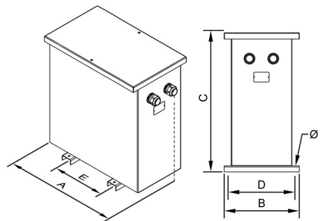
Dimensiones (AxBxCxDxE): 1050x900x1370x714x485 mm 18Ø
