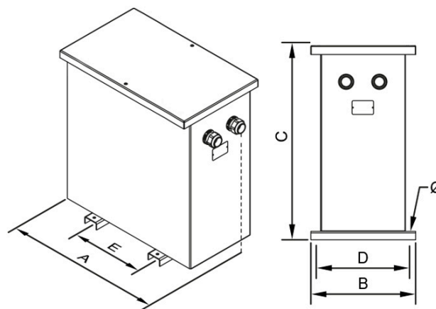
Dimensiones (AxBxCxDxE): 694x413x764x370x350 mm 11Ø
