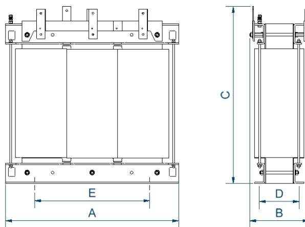
Dimensiones (AxBxCxDxE): 1300x550x1350x460x800 mm 17
