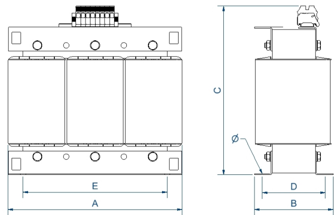
Dimensiones (AxBxCxDxE): 420x190x419x156x350 mm 11
