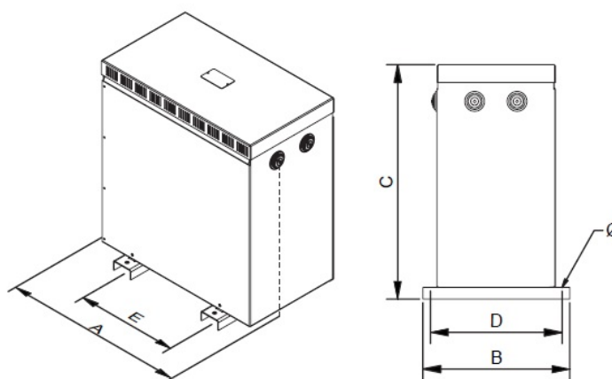
Dimensions (AxBxCxDxE): 315x230x315x205x200 mm 6Ø
