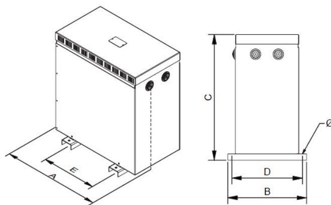
Dimensiones (AxBxCxDxE): 597x415x710x375x350 mm 12Ø
