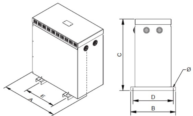
Dimensiones (AxBxCxDxE): 795x550x970x500x415 mm 12Ø
