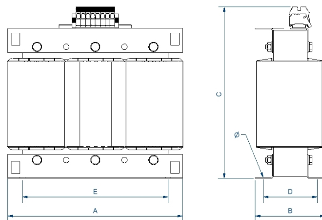
Dimensiones (AxBxCxDxE): 330x154x303x145x250 mm 9Ø
