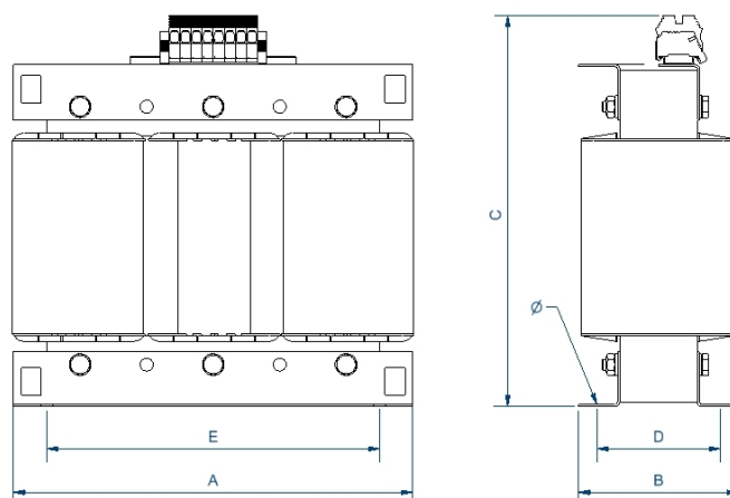
Dimensions (AxBxCxDxE): 330x154x303x145x250 mm 9Ø
