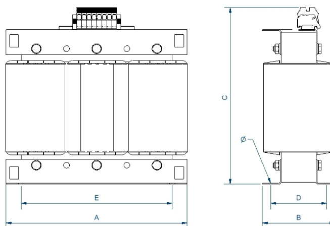
Dimensions (AxBxCxDxE): 330x164x303x155x250 mm 9Ø
