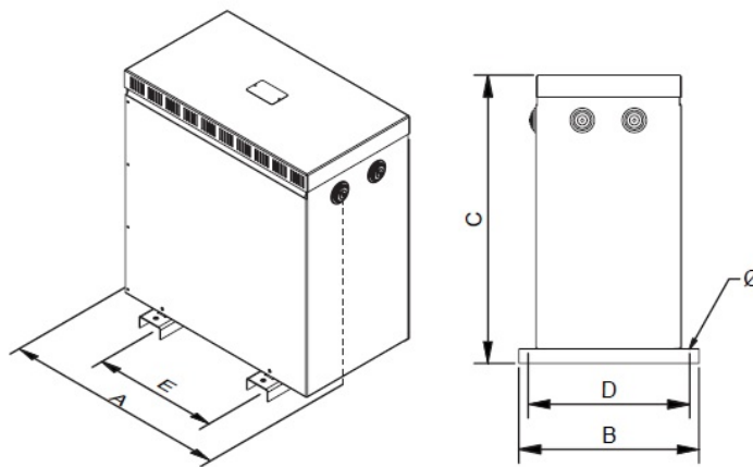
Dimensiones (AxBxCxDxE): 240x190x250x180x150 mm 6∅
