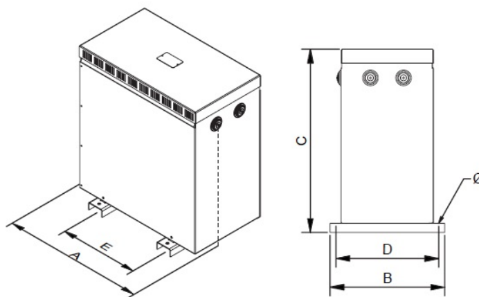
Dimensiones (AxBxCxDxE): 385x260x384x245x250 mm 6∅
