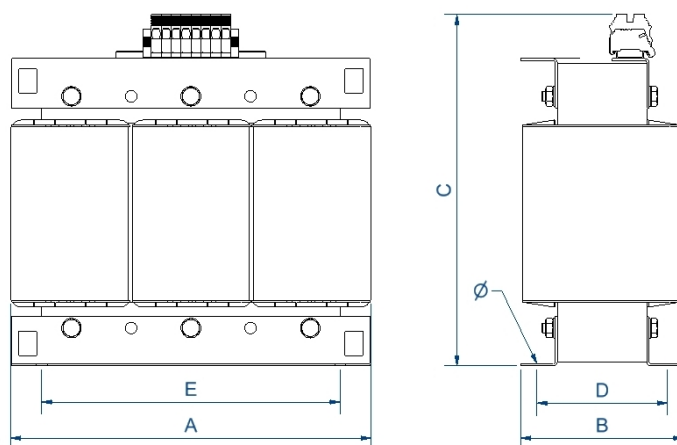
Dimensiones (AxBxCxDxE): 180x84x203x66x150 mm 6
