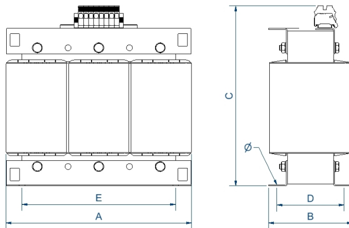
Dimensiones (AxBxCxDxE): 240x108x253x104x200 mm 9
