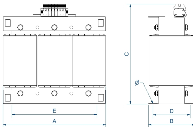
Dimensiones (AxBxCxDxE): 240x145x253x125x200 mm 9Ø
