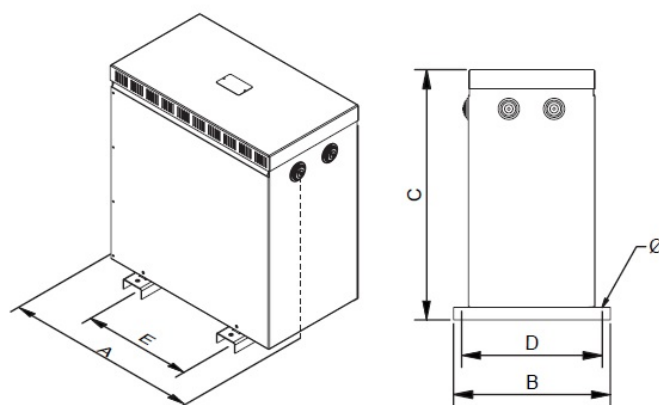
Dimensiones (AxBxCxDxE): 380x260x384x245x250 mm 6Ø
