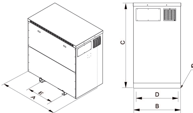
Dimensions (AxBxCxDxE): 1812x985x1791x900x800 mm 20Ø
