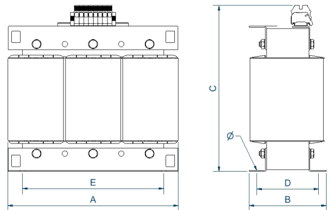
Dimensiones (AxBxCxDxE): 480x254x465x168x400 mm 110°
