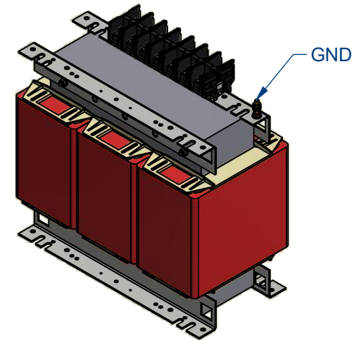
AUTW80 Enclosure ( 1/15 )
