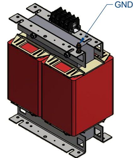
TKW12,5 Enclosure ( 1/18 )
