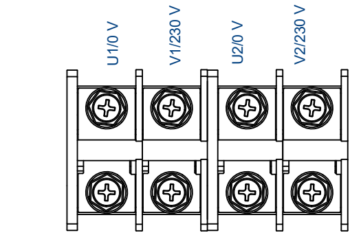
Connexion ( 1/2 )
