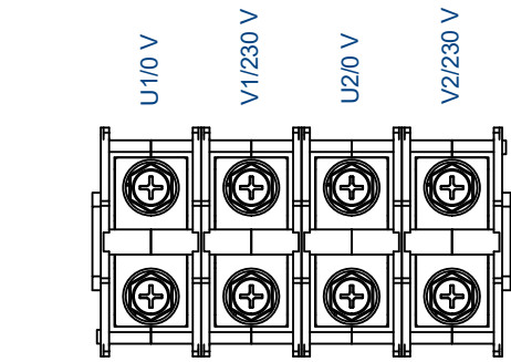
Connexion ( 1/3 )
